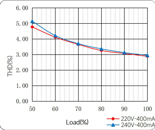
Зависимость полного гармонического искажения от нагрузки
